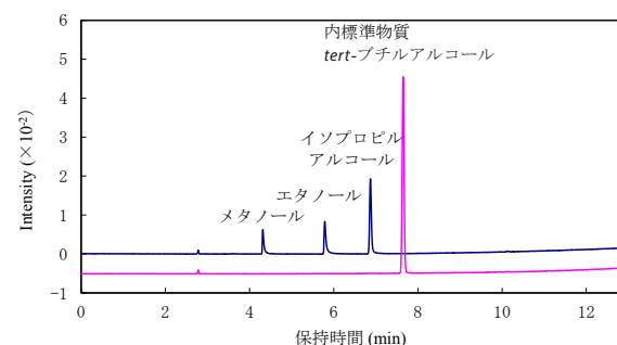
アルコール成分のクロマトグラム
