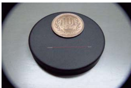
コンタクトチェッカープローブピン (φ0.09mm×30mm)
