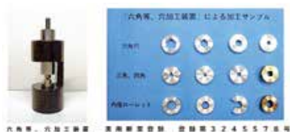
六角等穴加工治具
