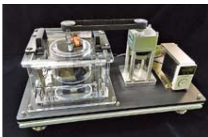
テイラークエット装置
