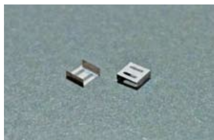
板厚5μmの精密抜き曲げ加工 (スリット幅0.5mm)
