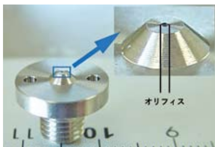
オリフィス 材質：SUS304
