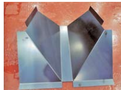
SS400 3.2mm板を ベンダーにて複雑な曲げ加工
