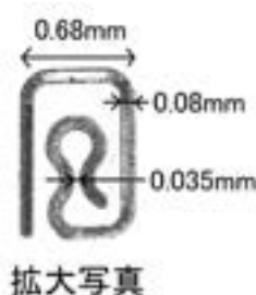
0.035mm細幅抜き加工 (重要箇所精度±3μm)
