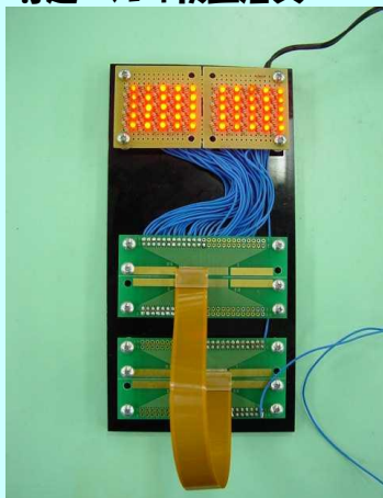
導通・ショート検査治具
