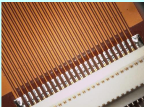
0.5mm pitchの50pinのFPC実装
