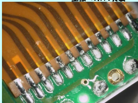
基板へのFPC実装
