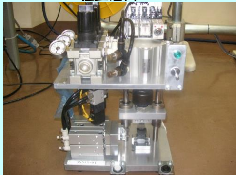
組立治具
