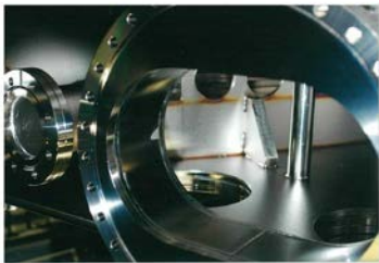
大型放射光施設ビームライン 真空チャンバー-SUS316L Size 1500x1200x H300
