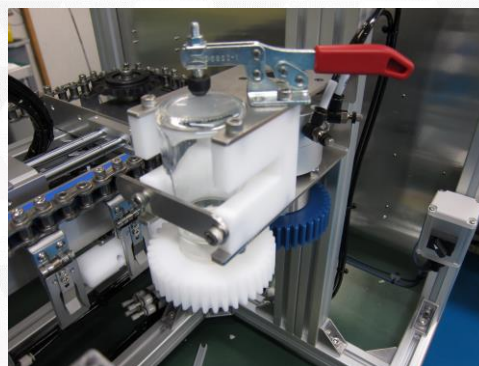
加工工程一例
