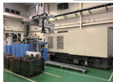
小さい部品から大型部品まで生産可能な成形機がラインナップ
