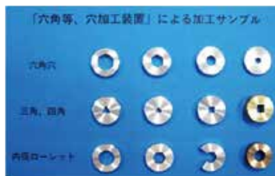
「六角等、穴加工装置」による加工サンプル 実用新案登録 登録第3 2 4 5 7 8号
