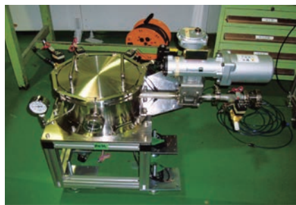
真空～加圧・加熱チャンバー (真空技術)
